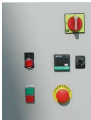
>Quadro elettrico
